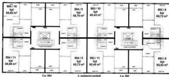
3. nadzemní podlaží
