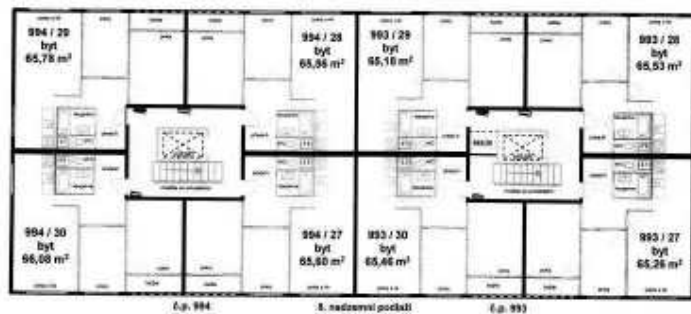
8. nadzemní podlaží
