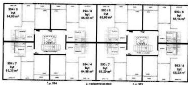
2. nadzemní podlaží
